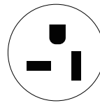
Nema 5-20
